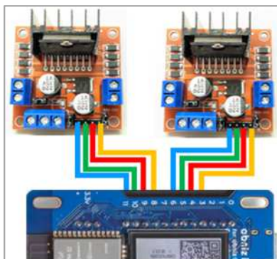
配線
